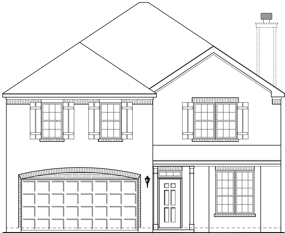
2412BF ELEVATION B
