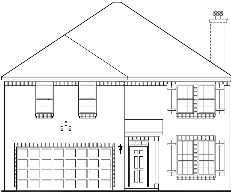
2412BF ELEVATION A
