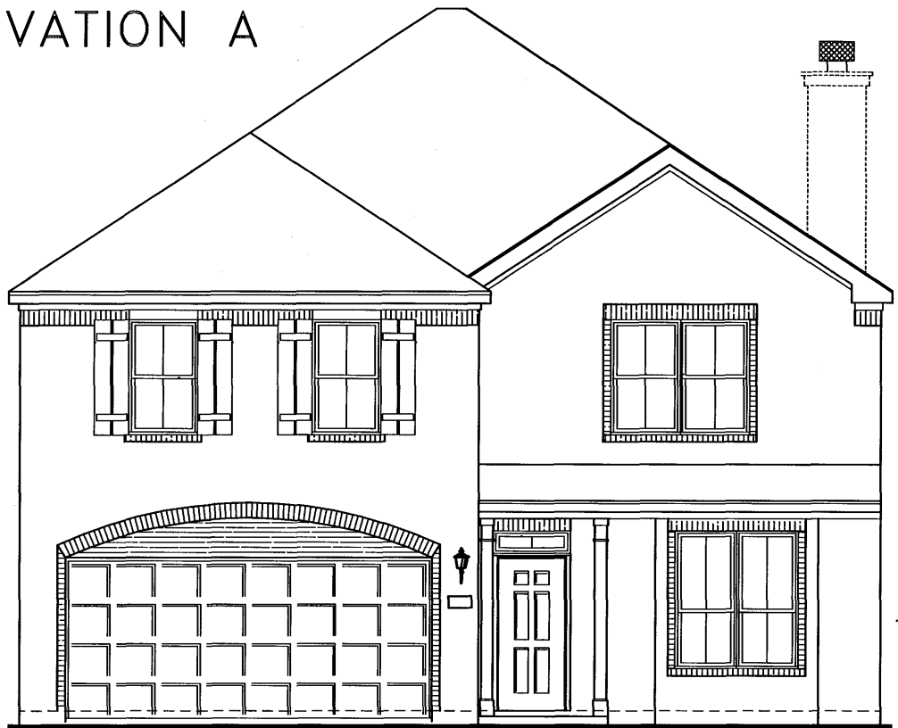
ELEVATION B
