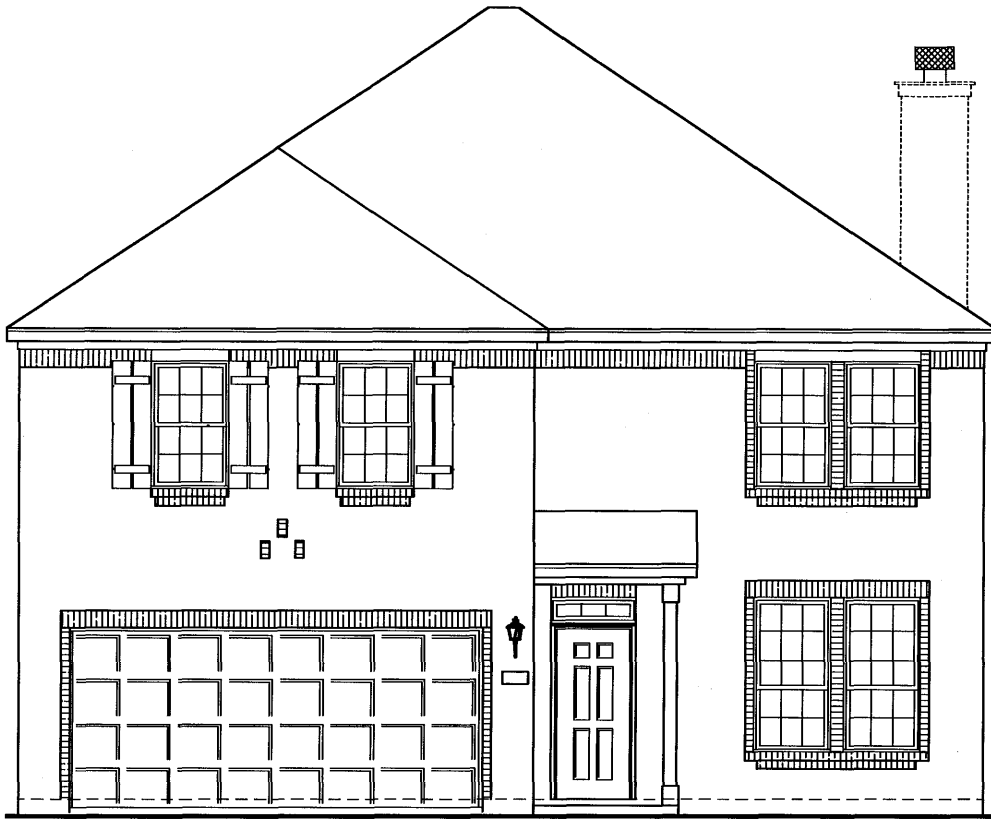
ELEVATION A
